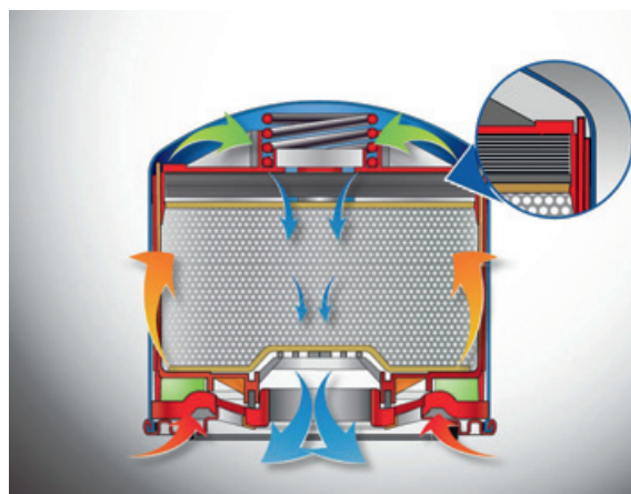
Ölfilter oben an der Lufttrocknerkartusche
